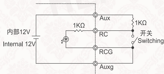
连接方法 Connection Method
