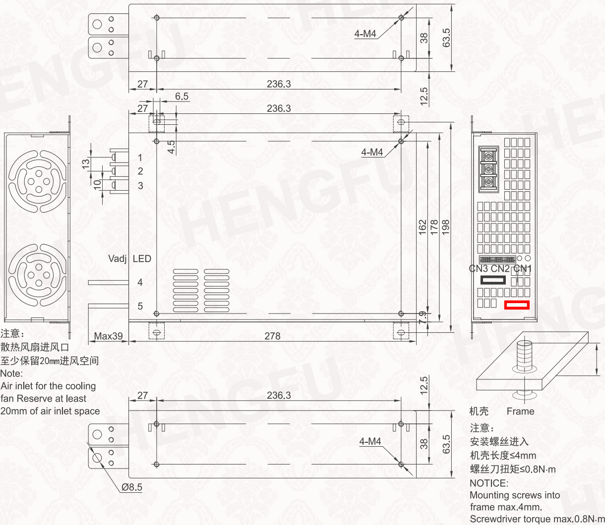
HF3000W-SCN-*** 13P+2输出输出安装图
