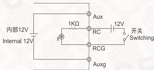
C: 用内部12V辅助输出 Using internal 12V auxiliary output
